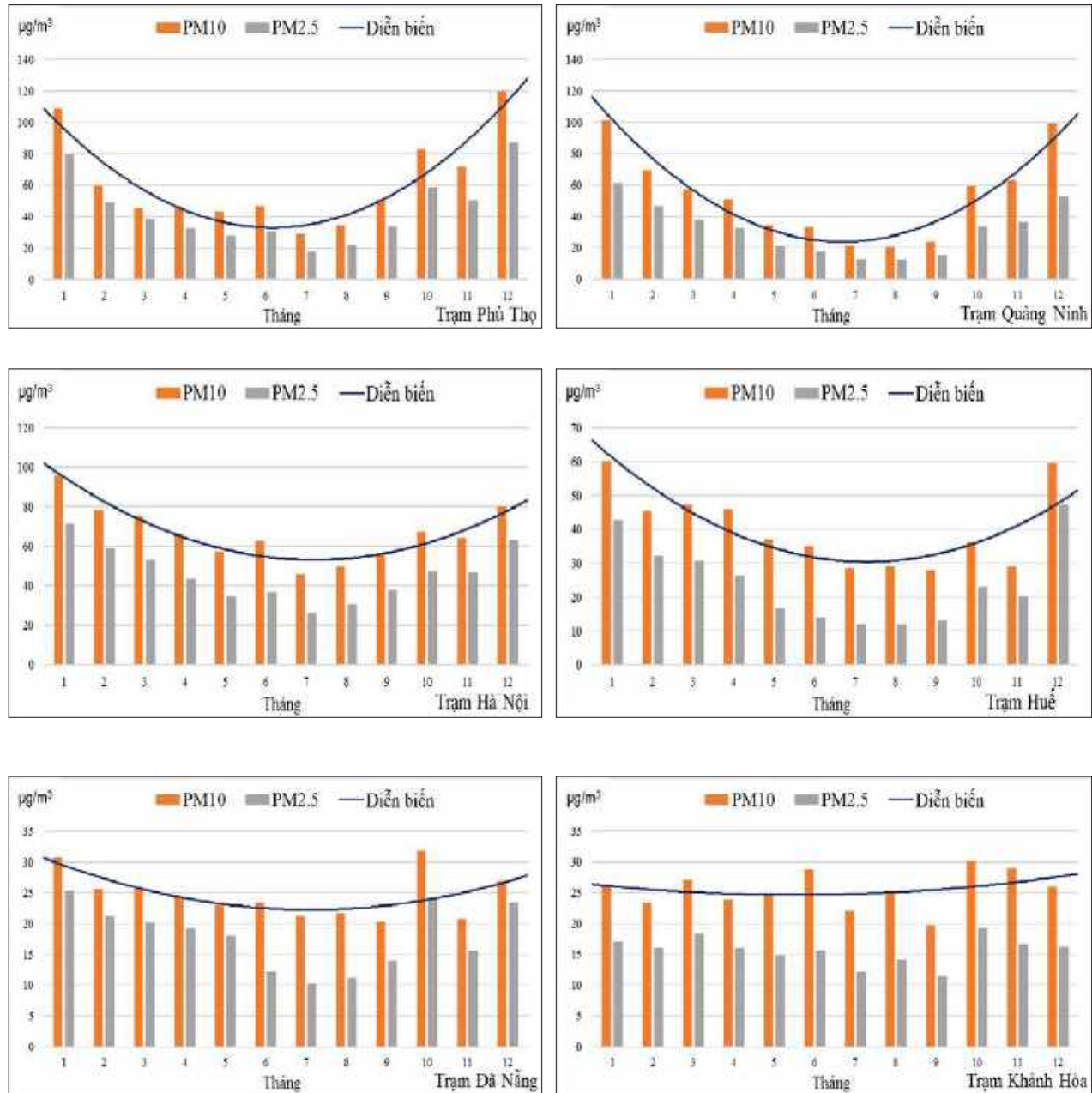
Biểu đồ 5.2. Giá trị trung bình tháng (tính qua các năm) của \text{PM}_{10} và \text{PM}_{2,5} tại các trạm quan trắc không khí tự động
