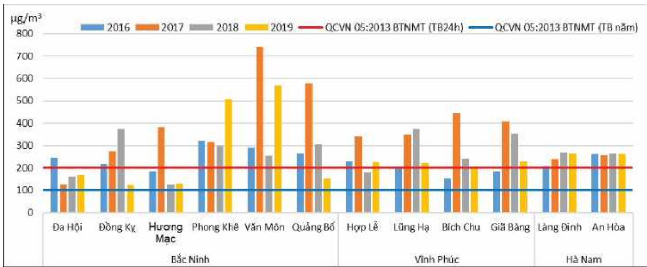
Biểu đồ 5.11. Diễn biến giá trị thông số TSP trong không khí tại một số làng nghề giai đoạn 2016 - 2019
