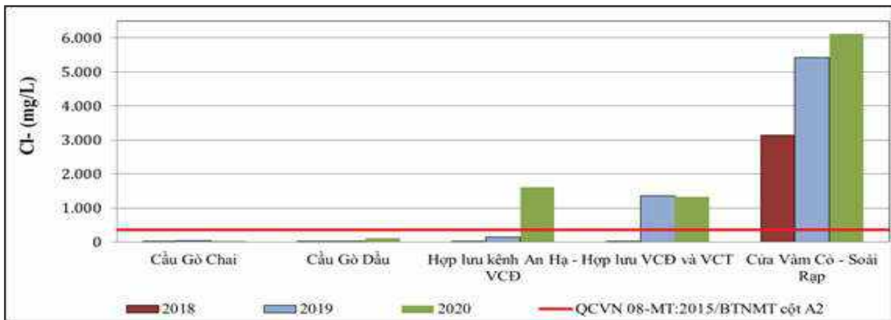
Biểu đồ 4.29. Diễn biến giá trị clorua trên sông Vàm Cỏ giai đoạn 2018 - 2020 Nguồn: Tổng hợp từ số liệu quan trắc của Tổng cục Môi trường
