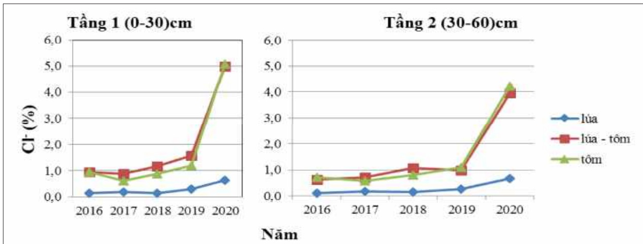
Biểu đồ 6.14. Diễn biến hàm lượng clorua trong đất mặn vùng đồng bằng sông Cửu Long giai đoạn 2016 - 2020
