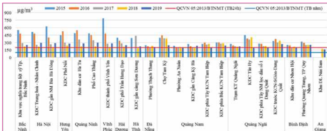
Biểu đồ 5.1. Diễn biến giá trị thông số TSP tại một số khu vực dân cư giai đoạn 2015 - 2019
