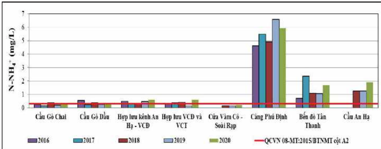
Biểu đồ 4.28. Diễn biến giá trị amoni trên sông Vàm Cỏ giai đoạn 2016 - 2020 Nguồn: Tổng hợp từ số liệu quan trắc của Tổng cục Môi trường
