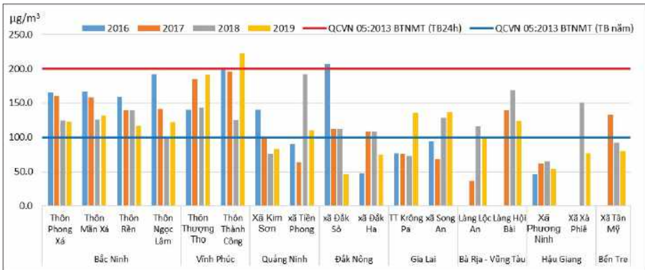
Biểu đồ 5.12. Diễn biến giá trị thông số TSP tại một số vùng nông thôn giai đoạn 2016 - 2019
